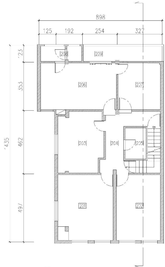
2 2樓平面圖 scale: 1/100
