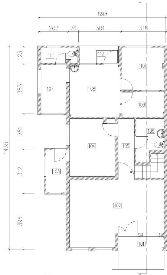
1 1樓平面圖 scale: 1/100
