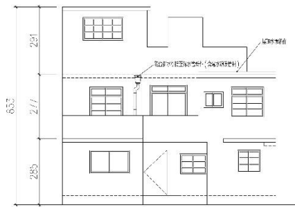
2 側立面圖 scale: 1/100
